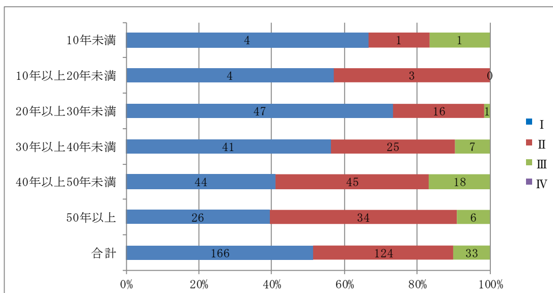
図 5-2 診断区分と建設経過年数
