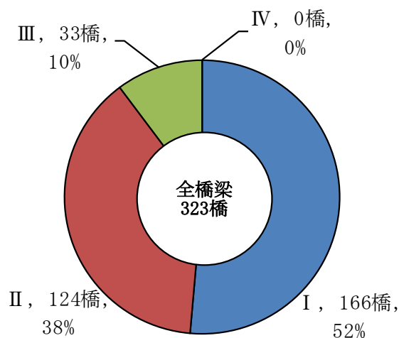
図 5-1 定期点検結果に基づく健全性
