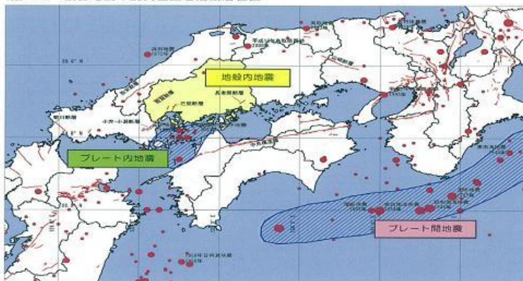
図－2 被害地震の震央位置と活断層位置
