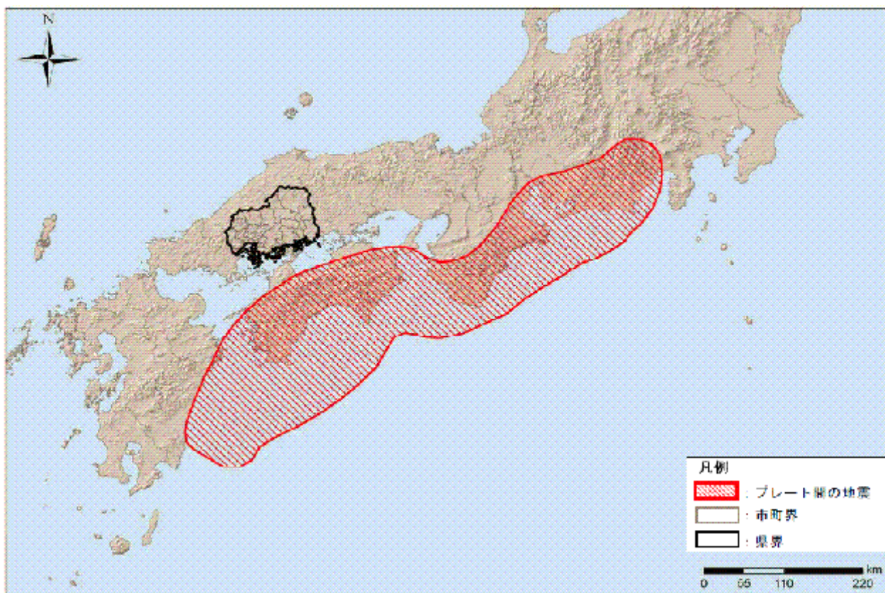
図一 1 想定地震位置図（南海トラフ巨大地震）
